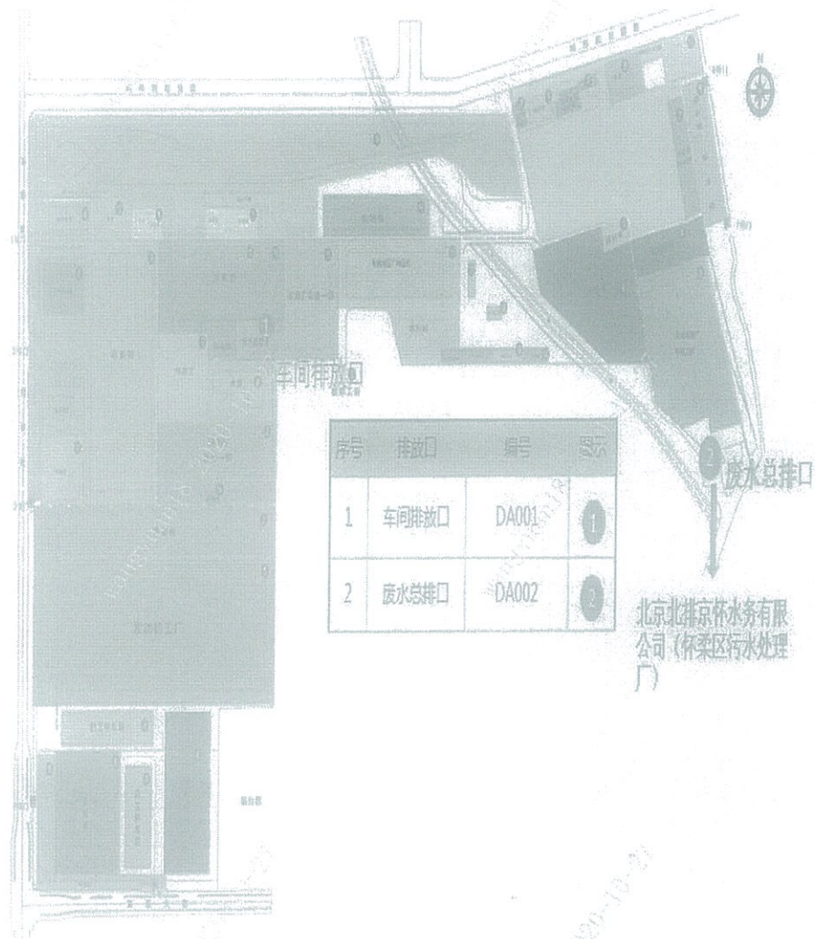
图 福戴一工厂废水排放口平面图 - 主要排放口(2个, 共2个)
